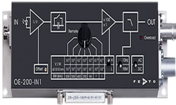
광전변환장치
