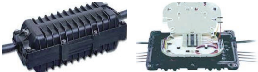
<광접속함체>
