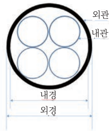
〈통신용 COD(Cable Optical Duct)관〉
